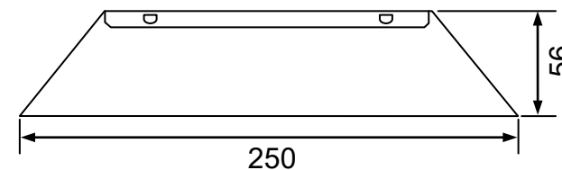
尺寸: 250*108*56mm
