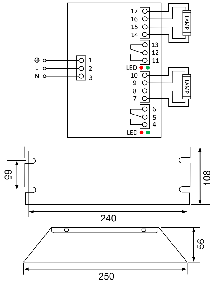
尺寸: 250*108*56mm
